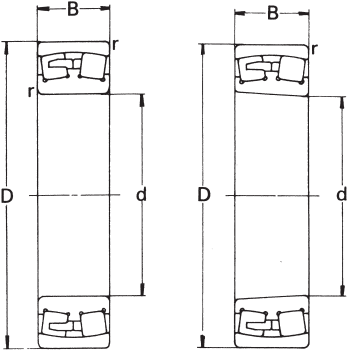
239 圓柱孔
