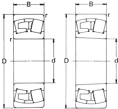
223R 圓柱孔
