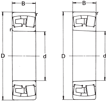
222 圓柱孔
