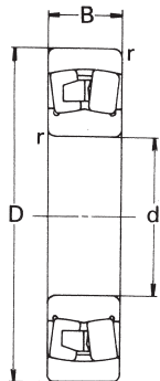
213 圓柱孔
