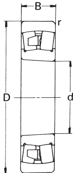
213K 圓錐孔 錐度 1 : 12
