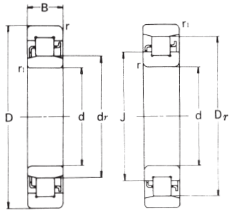
NU2 圓柱孔
