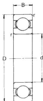
開放形
