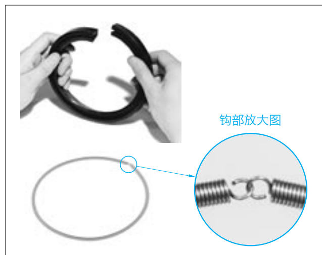
〈图-19.〉 MG型油封
