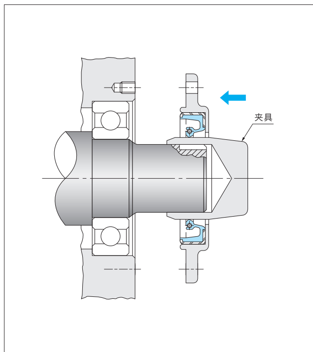
〈图-18.〉插入轴内的方法
