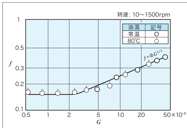
〈图-2.〉旋转用油封油封的摩擦特性 ( f \sim G 特性)
