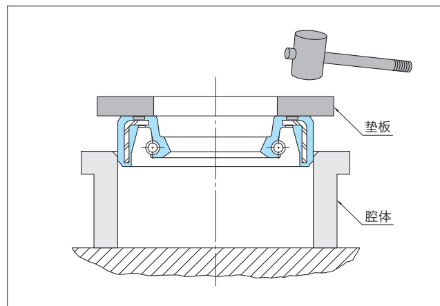
《图-8.》无法用压力机压入时的示例
