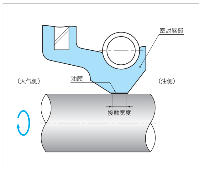
〈图-1.〉油封装上的状态
