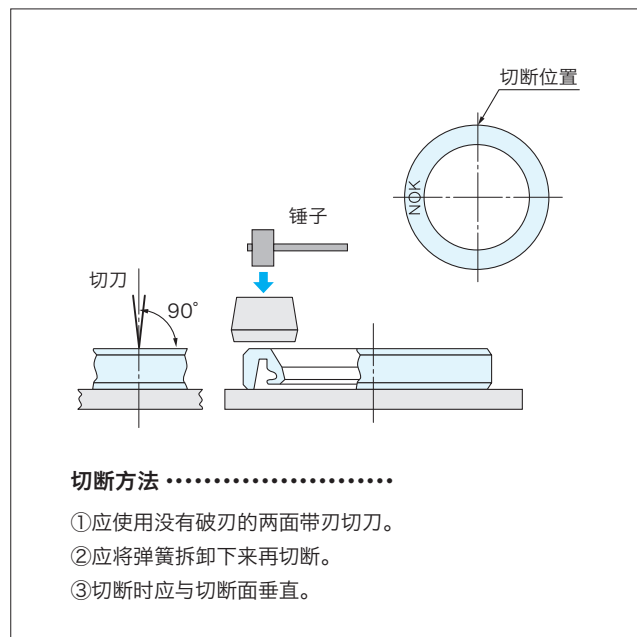
〈图-20.〉 MG 型油封的切断方法
