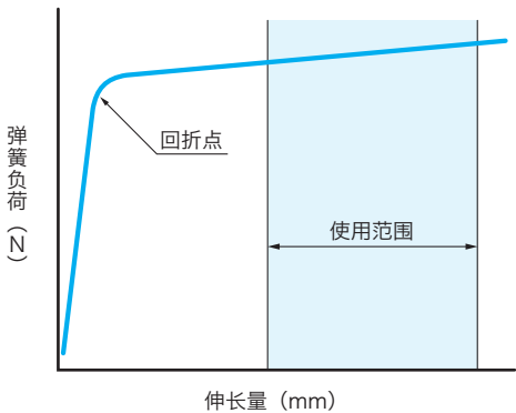
〈图-2.〉油封所使用的弹簧的特性
