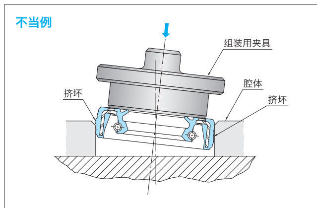
《图-7.》倾斜压入例
