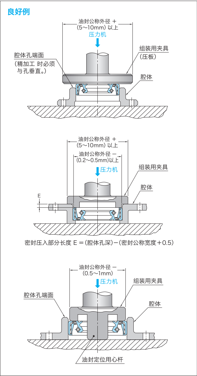
《图-5.》组装夹具使用例（配合部分为橡胶或金属均适用）
