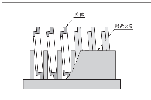
〈图-1〉腔体的運搬治具
