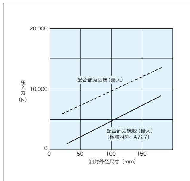
《图-10.》压入力的参考值 (100mm/min 参考)
