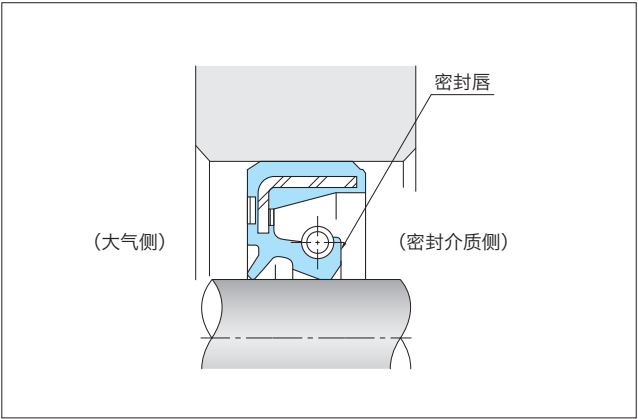
《图-4.》油封的方向
