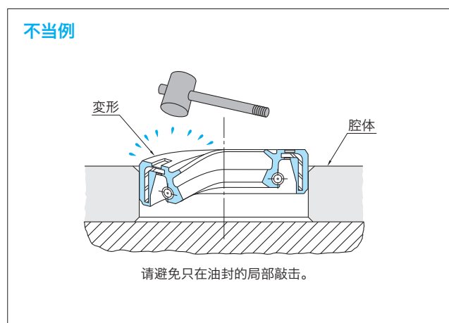
《图-9.》用锤压入不当例
